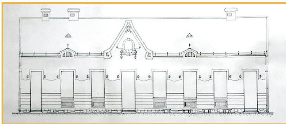
Část z výkresů na přístavbu „spolkové místnosti“, 1911
